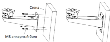
Рисунок 2-1 Установка кронштейна
