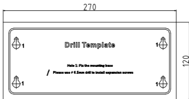
Рисунок 2-7 Шаблон крепления
